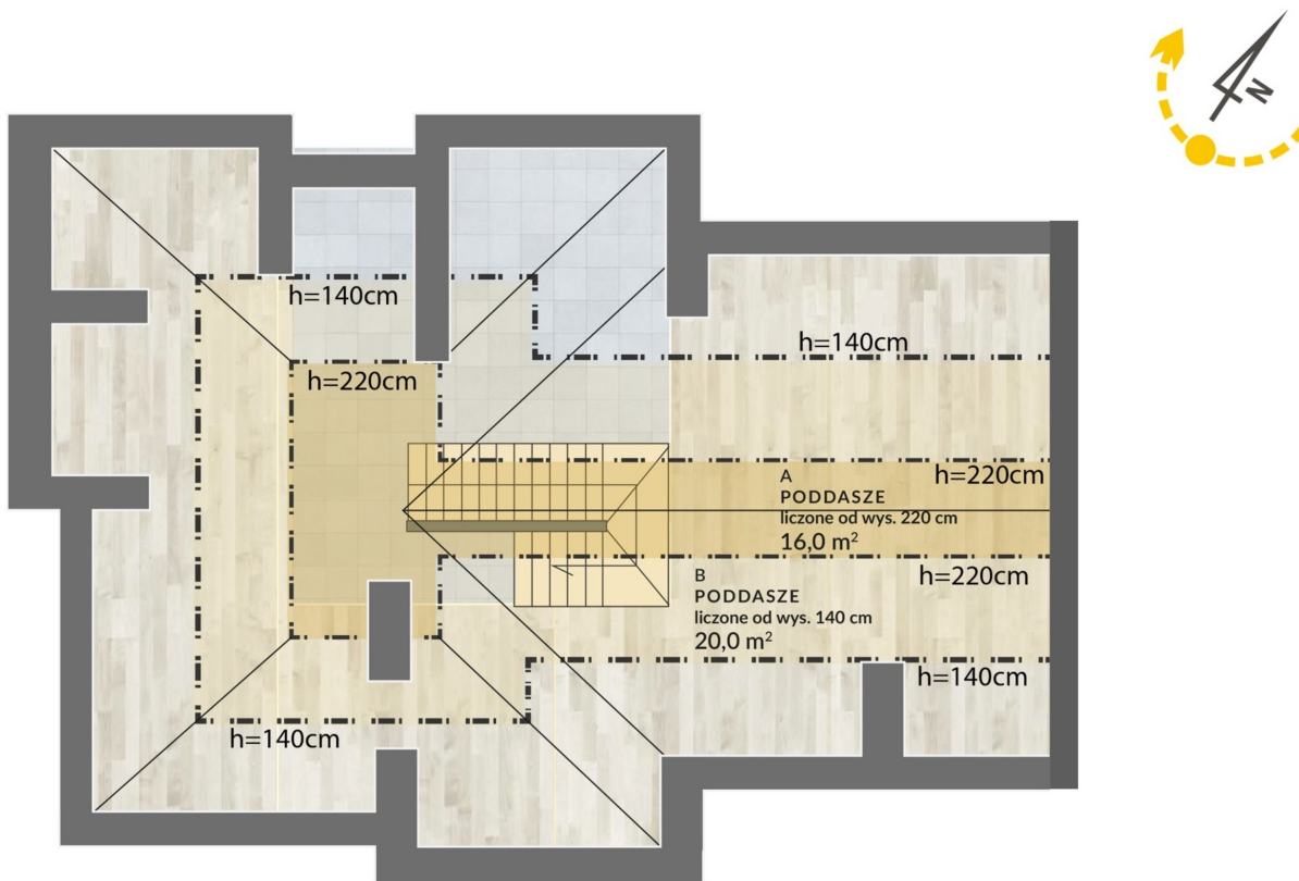
Rzut poddasza
