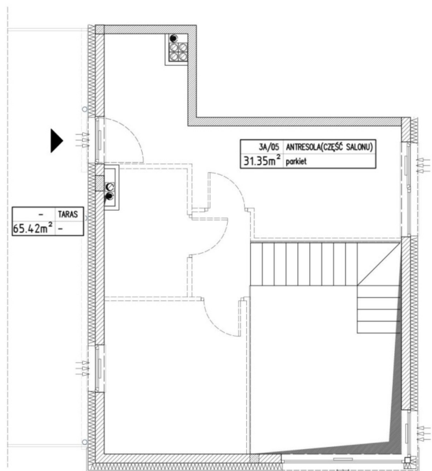
RZUT ANTRESOLI
