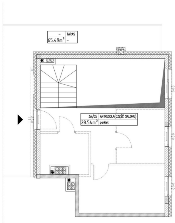
RZUT ANTRESOLI
